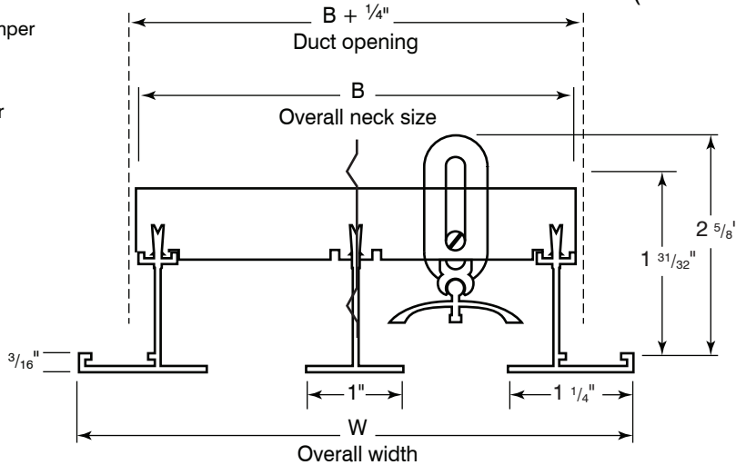
ALS50 / ALS57 (ALS27 two slots shown here)
