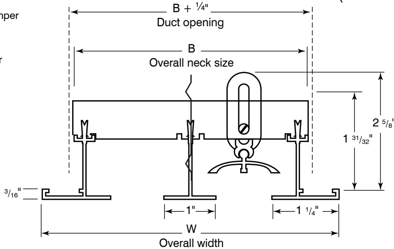
ALS40 / ALS47 (ALS27 two slots shown here)
